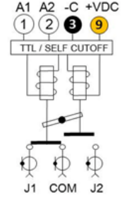
TTL和自切断 (仅闭锁)
