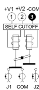
自切断 (仅闭锁)
