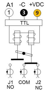
失效保护 TTL
