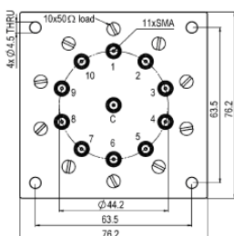
机械图纸 (单位: mm) H = 50 (max) (标准) = 60 (max) (带TTL) = 65 (max) (带指示器时)
