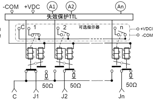
每个未使用位置为常开 图2
