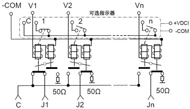
每个未使用位置为常开 图1
